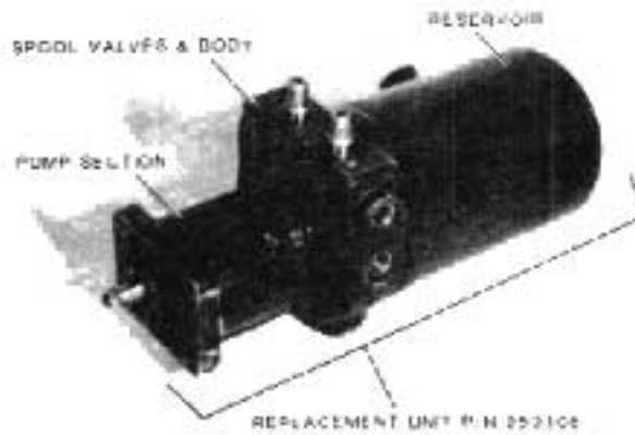
FIG. 1. Dual Hydraulic Unit - VIN 81 & 91-20RG01
